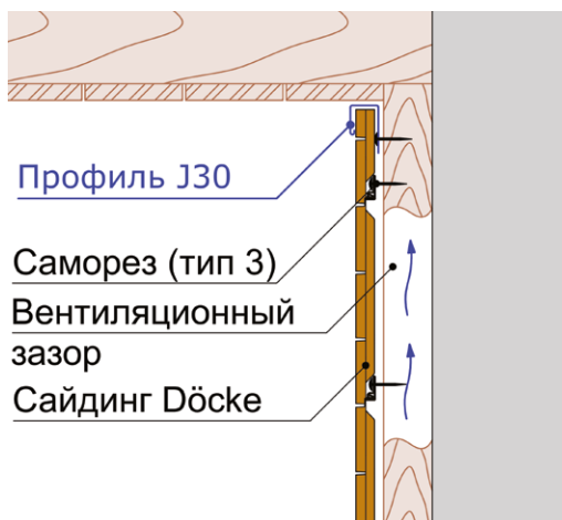
Рис. 20 Примыкание сайдинга Döcke LUX под камень к горизонтальной поверхности.
