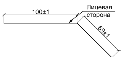
Планка карнизная ПКД-100х69х2000
