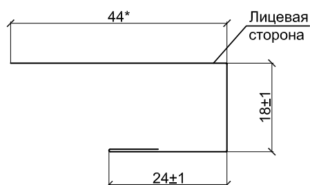
Планка J-профиль ПЈ-24х18х2000 (3000)
