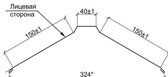
Планка конька плоского ПКП-150x150x2000
