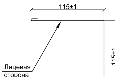
Планка угла наружного ПУВ-115х115х2000
