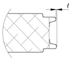
Рисунок 15 – Схема измерения смещения продольных кромок
