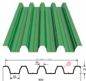
Профилированный лист H-75x750-A Толщина материала 0.65 - 1.0 мм
