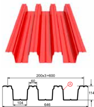
Профилированный лист H-114x600-A Толщина материала 0.7 - 1.0 мм
