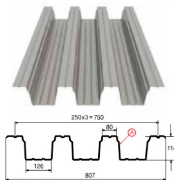
Профилированный лист H-114x750-A Толщина материала 0.7 - 1.0 мм
