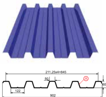
Профилированный лист H-60x845-A Толщина материала 0.5 - 1.0 мм
